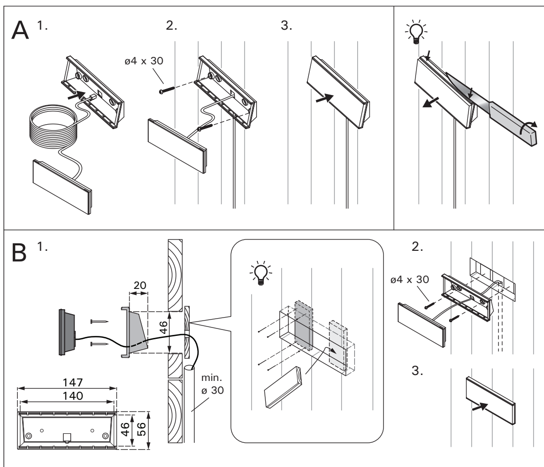
8. zīmējums. Vadības panela piestiprināšana 8 pav. Valdymo pulto instaliavimas
